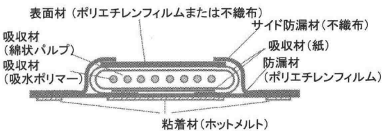
図2. 試料の素材と構成
